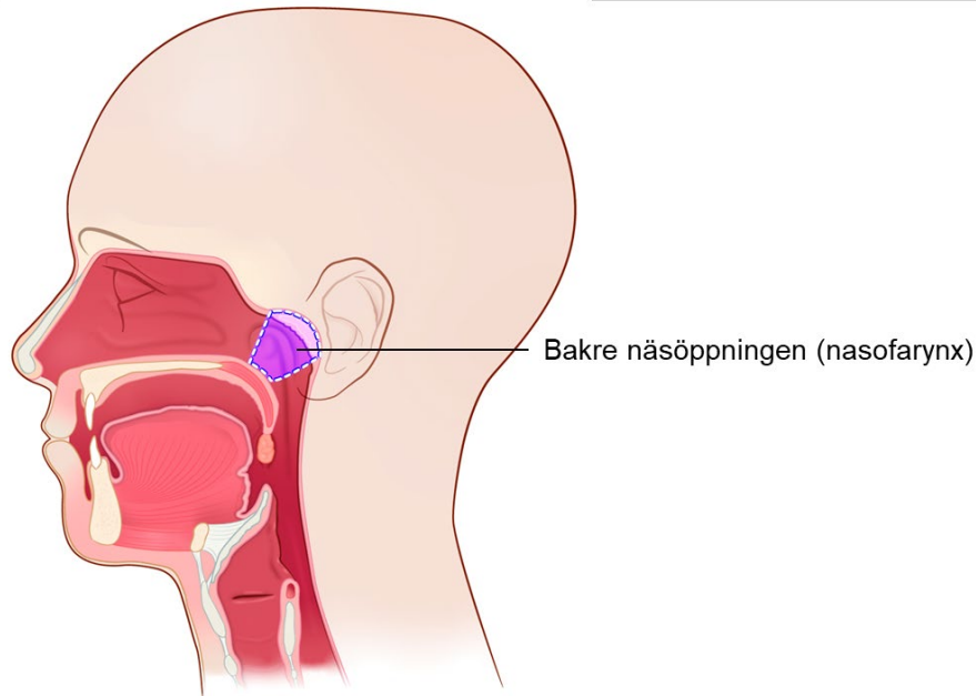
Bakre näsöppningen
