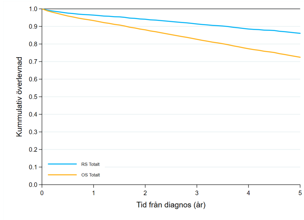
Figur 13. Observerad (OS) och relativ (RS) 3- och 5-årsöverlevnad, diagnosår 2007–2023.
