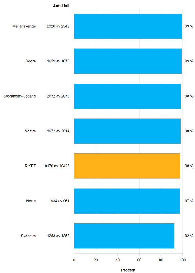
Figur 3. Täckningsgrad (per region och för riket) för hela perioden 2007–2023.
