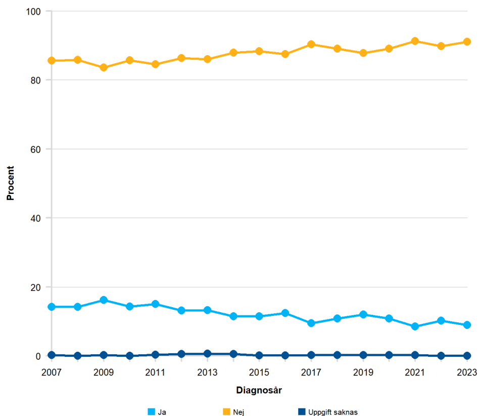
Figur 2. Andelen patienter med behov av behandling (Ja) eller inte behov av behandling (Nej) vid diagnos av KLL i Sverige 2007–2023, med förändring över tid.
