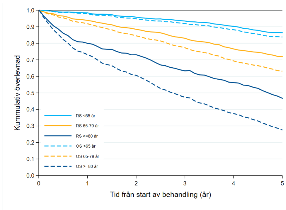
Figur 15. Total överlevnad (OS=overall survival) och relativ överlevnad (RS=relative survival) efter start av behandling 2007–2023 (n= 2792), uppdelat på tre ålderskategorier (<65 år, 65-79 år samt => 80 år vid start av behandling).
