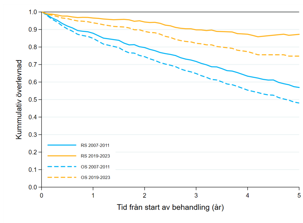
Figur 16. Total överlevnad (OS=overall survival) och relativ överlevnad (RS=relative survival) för patienter med start av behandling 2007-2011 och 2019-2023.
