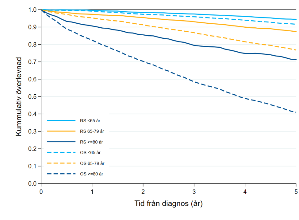
Figur 14. Total överlevnad (OS=overall survival) och relativ överlevnad (RS=relative survival) från diagnos för alla patienter med diagnos 2007–2023 ( n=10\,070 ) uppdelat på tre ålderskategorier (<65 år, 65-79 år samt \geq 80 år).
