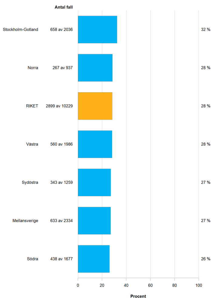
Figur 1. Andelen patienter <65 år vid diagnos fördelat på sjukvårdsregion, 2007–2023.
