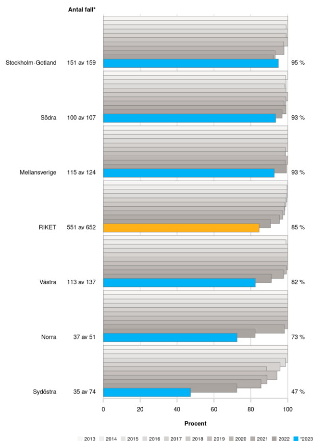
Figur 4. Täckningsgraden (per region och riket) redovisad per år under perioden 2013–2023.
